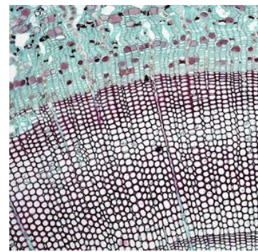
les cellules
